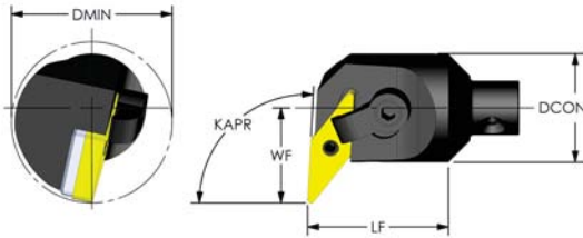
Negative 35° Diamond (KAPR: 93°) Profiling
