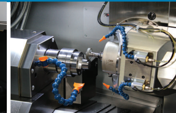
OD Taper Grinding
