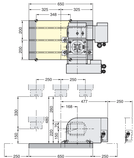
5AX-DD200
